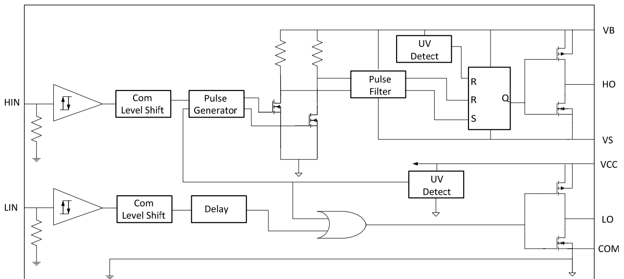
图 3. 功能框图
