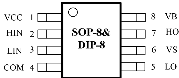
图2. 管脚分布
